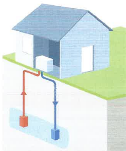
Principe de la géothermie sur nappe : échangeurs ouverts, pompe à chaleur eau-eau.
