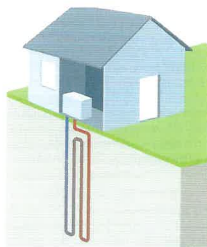
Principe de la géothermie sur sonde : échangeurs fermés, pompe à chaleur terre-eau.
